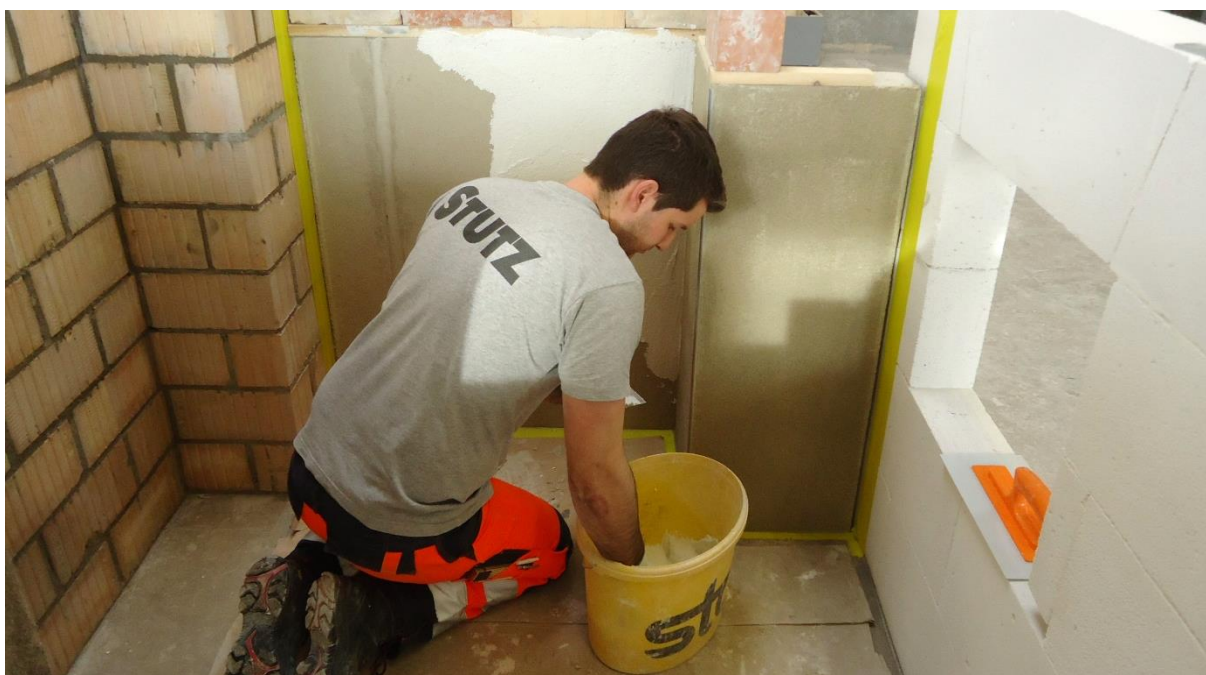
Mauerwerke aus verschiedenen Steintypen und Verputzarbeiten (Foto: BVKSG)
