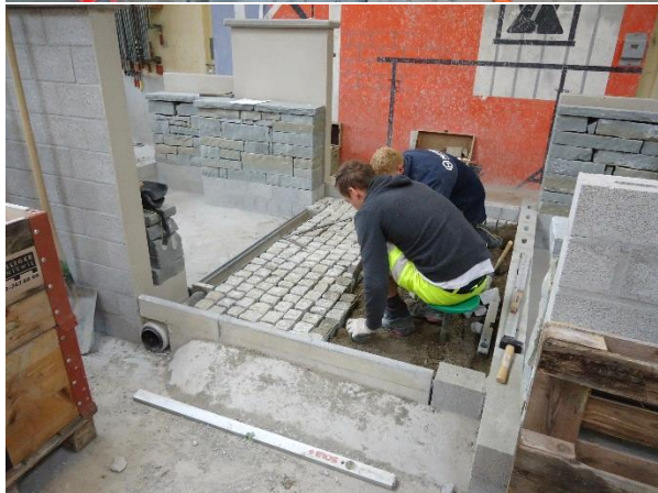
Natursteinwerk, Pflasterungen und Kanalisation (Fotos: BVKSG)
